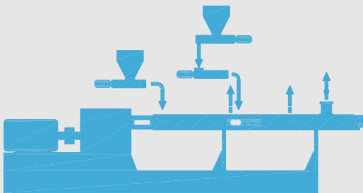
母料制备
