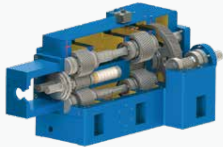
双螺杆传动箱
