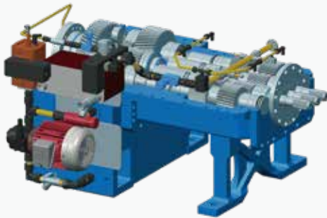
三螺杆传动箱
