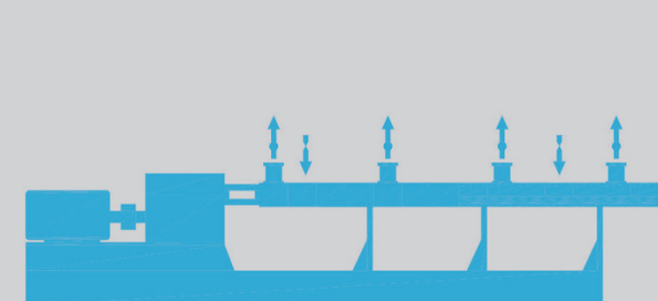
Изображение4 Реактивная экструзия и дегазация
