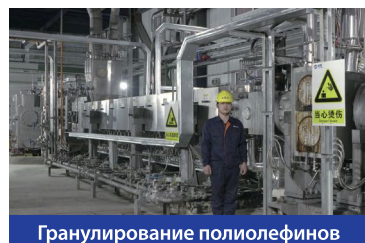
Гранулирование полиолефинов
